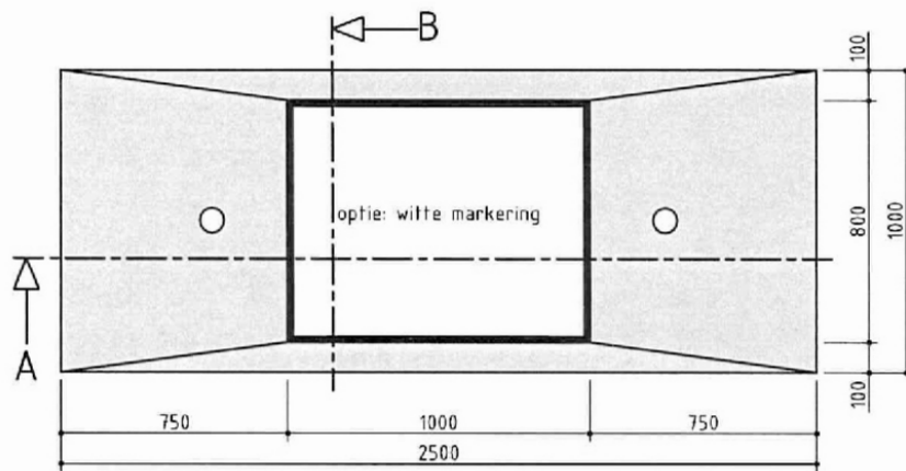
AANZICHT STORTZIJDE
