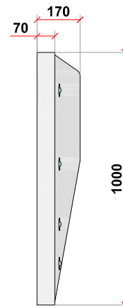
Zijaanzicht
