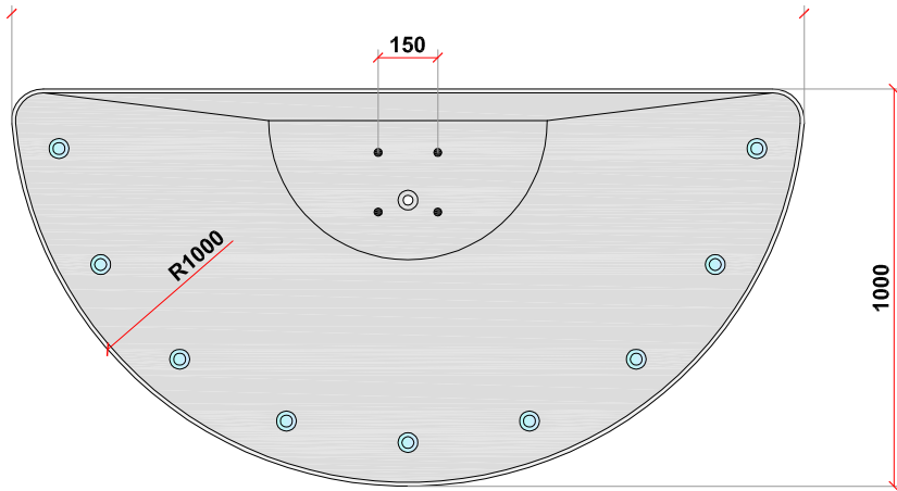
Bovenaanzicht
