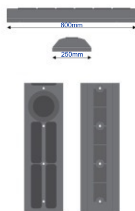
tussenstuk zonder half ronde uitsparing art. 641-111
