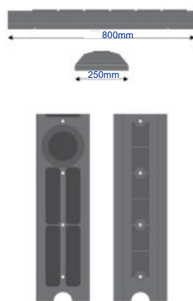
tussenstuk met half ronde uitsparing art. 641-110
