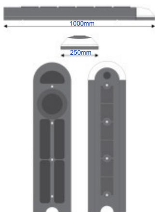
kop/eindstuk met half ronde uitsparing art. 641-104
