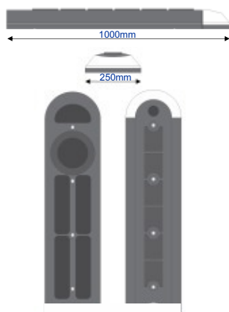
kop/eindstuk zonder half ronde uitsparing art. 641-113
