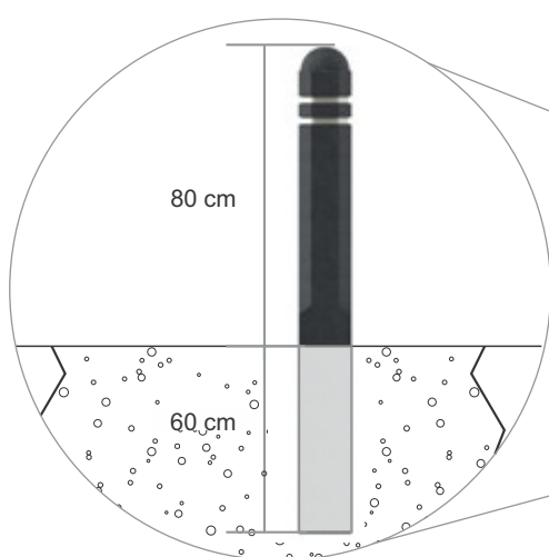
Sokkel voor wegneembare paal
